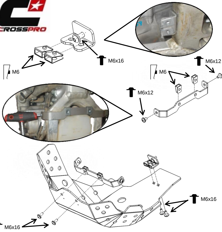
Instrução de Montagem / Assembly Sequence
